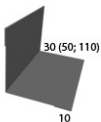
Планка угла внутреннего простая
