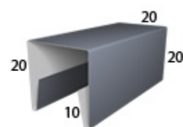
Планка П-образная заборная 20
