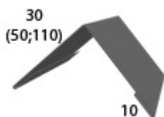
Планка угла внешнего простая
