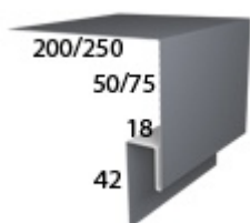
Околооконная планка сложная (200x50; 200x75; 250x50; 250x75)
