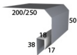
Околооконная планка сложная фигурная (200x50; 250x50)
