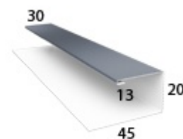
Планка завершающая сложная (П-образная планка)
