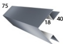
Планка угла внешнего сложная
