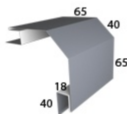
Планка угла внешнего сложная фигурная
