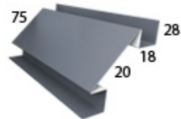
Планка угла внутреннего сложная
