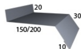
Отлив простой (150; 200)
