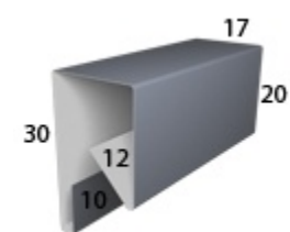
Планка П-образная заборная 17
