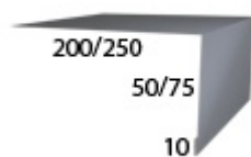
Околооконная планка простая (200x50; 200x75; 250x50; 250x75)
