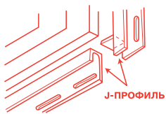
ЗАПАС В 6,4 ММ ДЛЯ РАСШИРЕНИЯ ПАНЕЛЕЙ
